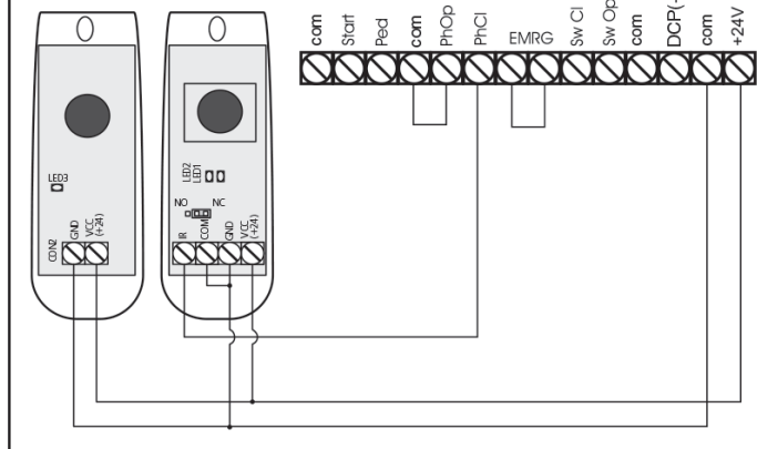
Подключение фотоэлементов на закрытие. При использовании фотоэлементов PhotoCell (DoorHan) установите джемпер в положение NC
