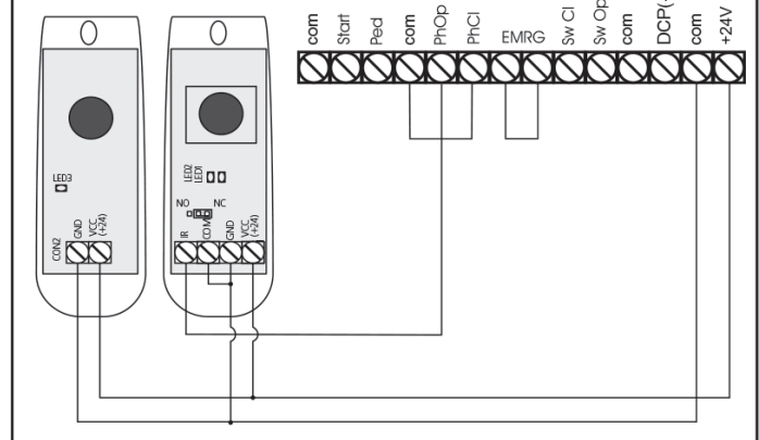
Подключение фотоэлементов на открытие. При использовании фотоэлементов PhotoCell (DoorHan) установите джемпер в положение NC
